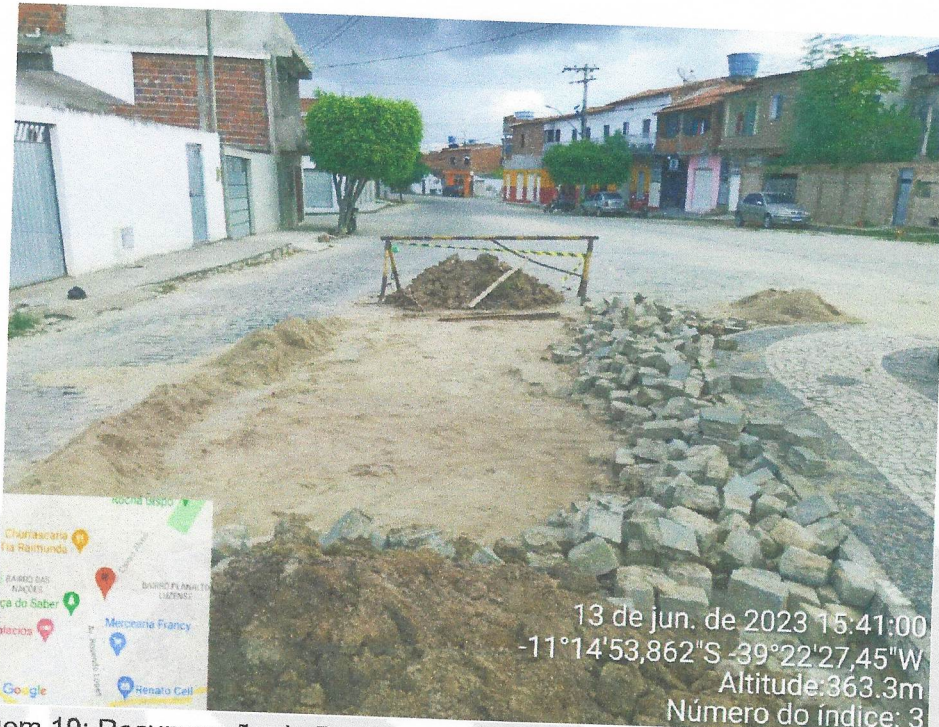
Imagem 19: Recuperação da Pavimentação em Paralelo na AV Castro Alves/Sede
