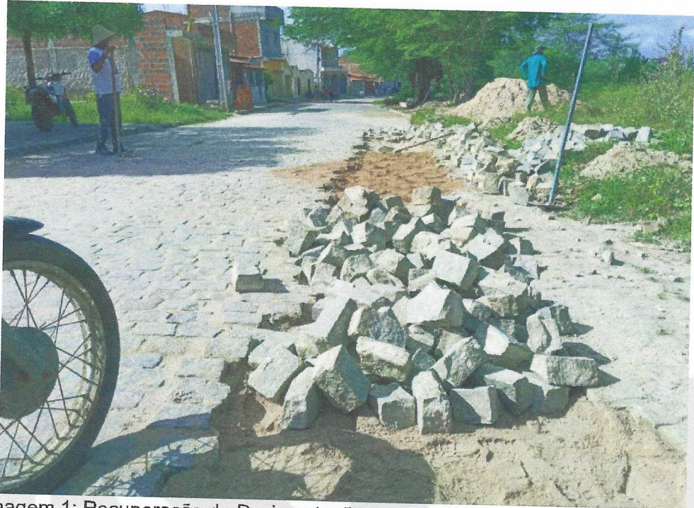
Imagem 1: Recuperação de Pavimentação em Paralelo na Rua J.J Seabra/Sede
